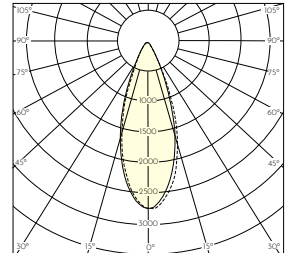
Curva fotometrica 36° 4000K 1270lm
