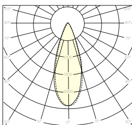
Curva fotométrica 36° 2700K 1140lm
