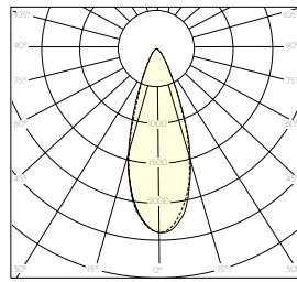
Curva fotométrica 36° 3000K 1170lm
