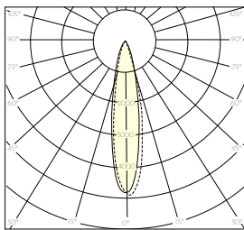
Curva fotométrica 24° 2700K 1140lm
