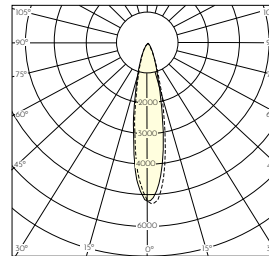
Curva fotometrica 24° 4000K 1270lm
