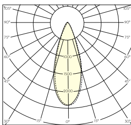
Curva fotometrica 36° 2700K 1140lm
