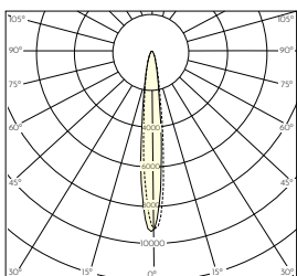
Curva fotometrica 12° 2700 K | 3000 K | 4000 K 970 lm | 1,140 lm | 1,140 lm
