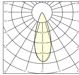
Curva fotometrica 36° 3000K 1170lm
