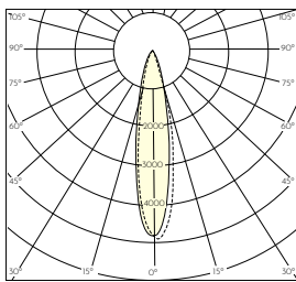
Curva fotometrica 24° 2700K 1140lm
