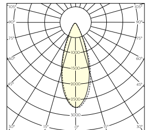
Curva fotometrica 36° 4000K 1270lm
