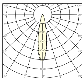
Curva fotometrica 24° 3000K 1170lm
