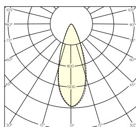
Curva fotométrica 36° 2700K 770lm
