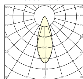
Curva fotométrica 36° 3000K 840lm
